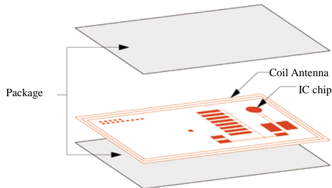
Fig. 3.7 RFID タグ構造
