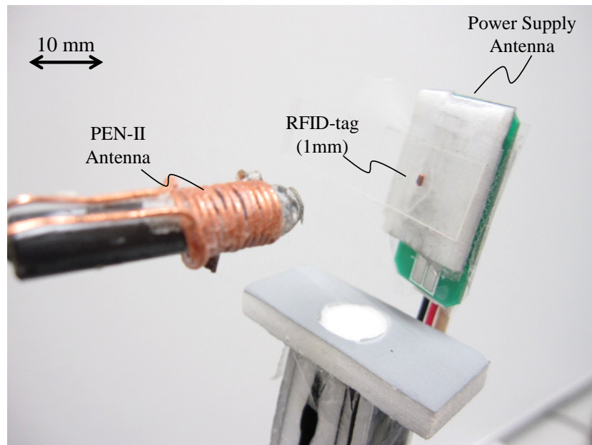
Fig. 3.40 PEN-II 型アンテナ特性検証の様子 (空气中)
