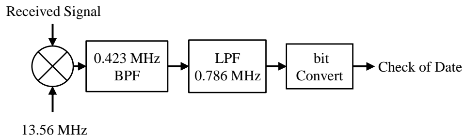
Fig. 3.33 複数 RFID タグ分離処理ブロックダイアグラム
