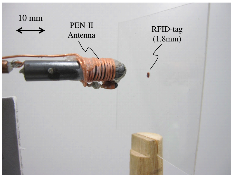
Fig. 3.27 RFID タグ 3 種類 ( 10 × 2.2 mm, 1.8 × 1 mm, 1 mm \phi ) の振幅測定
