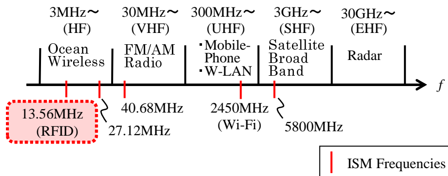
Fig. 3.3 無線通信に用いられる周波数帯域例
