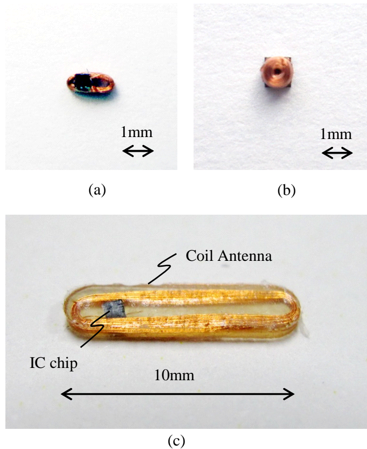
Fig. 3.8 大きさ異なるパッシブ型 RFID タグ : (a) 1.8 \times 1 \text{ mm} , (b) 1 \text{ mm}\phi , (c) 10 \times 2.2 \text{ mm}
